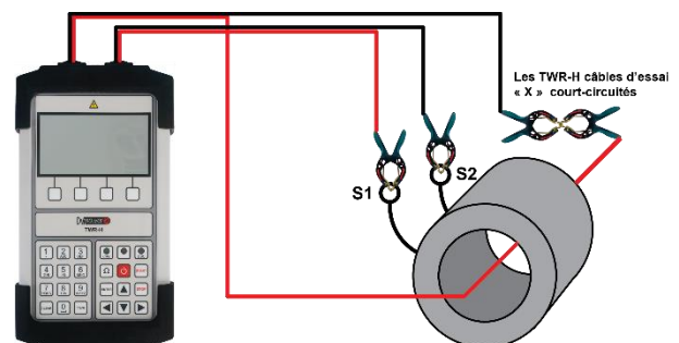
Raccordement de TWR-H à un transformateur de courant (TC) démonté
